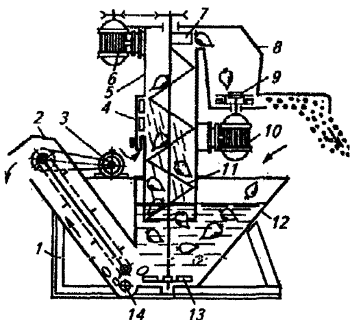
2.2.5 - rasm. IKM-F-10 rusumli ozuqalarni yuvgich maydalagich: 1-rama; 2-transportyor; 3,6 va 10-elektrodvigatel; 4-suv kollektori; 5-g'ilof; 7-uzatgich; 8-maydalagich korpusi; 9-maydalagich; 10-elekr dvigateli; 12-filtr; 13-nasos; 14-to'siq.
