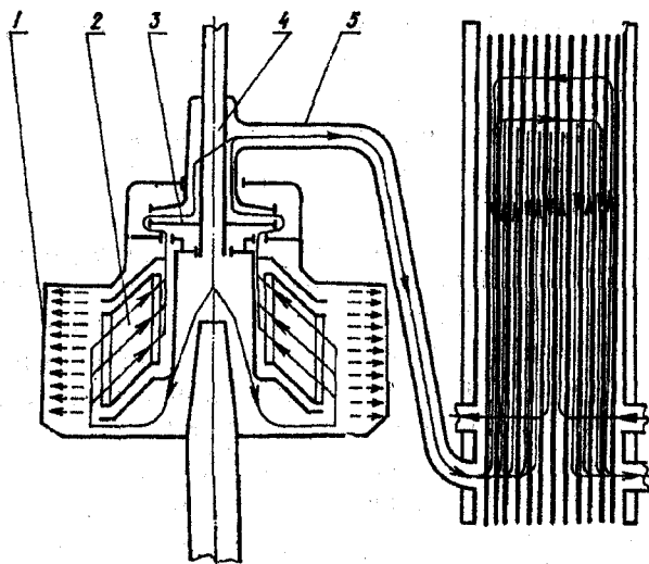
3.7.3-rasm. OM-1 sut tozalagich-sovitgichining ishlash sxemasi: 1-baraban korpusi; 2-barabandagi tarelkalararo bo'shliq; 3-chiqarish diski qurilmasi; 4- markaziy truba; 5- chiqarish trubasi.
