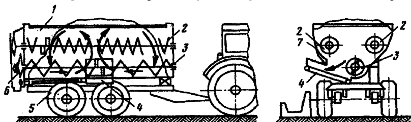
3.4.3-rasm. RSP-10 oзуqа tarqatgich sxemasi:
