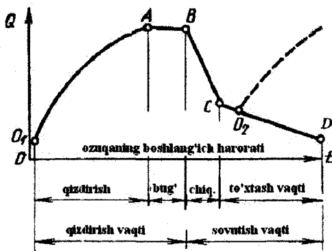
2.2.9-rasm. Bug‘latgichning ishlash grafi.
