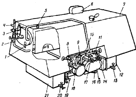
3.11.1-rasm. VDM-2 veterinariya dezenfeksiyalash mashinasi sxemasi: 1-yondiruvchi svecha; 2,8,11,13,14,17,19,20-ventillar; 3-forsunka; 4,9-shtutserlar; 5-qalquvchi datchik; 6-nazorat o'lchov asboblari shiti; 7-asosiy bak; 10-quyish shtutseri; 12-dezinfeksiyalovchi konsentratlar baki; 13-havo haydash kompressori (YAAZ-204); 16-havo so'rish shtutseri; 18-uyurmali nasos (VK2-26); 21-yoqilg'i baki.
