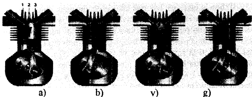
1.2.3 - rasm. To'rt taktli karbyuratorli ichki yonuv dvigatellarining ish sikli sxemasi: a -kiritish takti; b -siqish takti; v -ish bajarish takti; g -chiqarish takti. 1- kiritish klapani; 2- o't oldirish svechasi; 3- chiqarish klapani.
