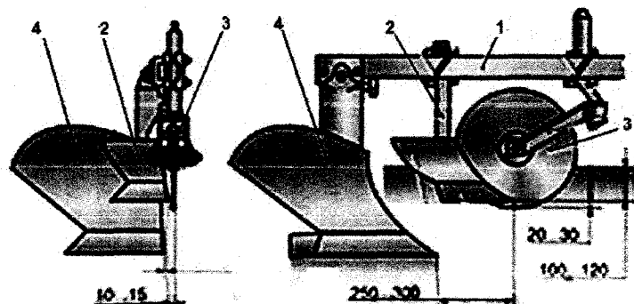
2.1.1 - rasm. Plug ishchi qismlarini joylashtirish sxemasi: 1-rama; 2-chimqirqar; 3-disklipichoq; 4-asosiy korpus.
