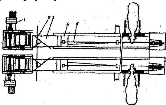
3.4.6-rasm. KLO-75 rusumidagi lentali ozuqa tarqatgichi: 1-yuritma; 2-to'xtatuvchi mexanizm; 3-lenta; 4-aravacha; 5-tortuvchi tros.
