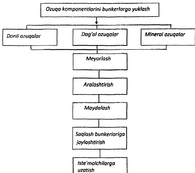
2.2.18-rasm. Omuxta yem tayyorlashning texnologik sxemasi.
