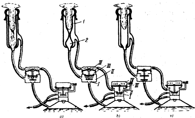
3.6.5-rasm. Uch taktli “Volga” sut sog‘ish apparatining ishlash sxemasi: a -so‘rish takti, b -siqish takti, v -dam olish takti; 1 -devorlararo kamera, 2 -so‘rish osti kamerasi; I - doimiy vakuum kamerasi, II , IV - o‘zgaruvchan bosim kameralari, III -atmosfera bosim kamerasi.
