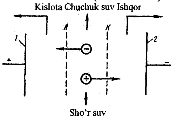
4.3.5-rasm. Elektrodializ qurilmasining sxemasi:
