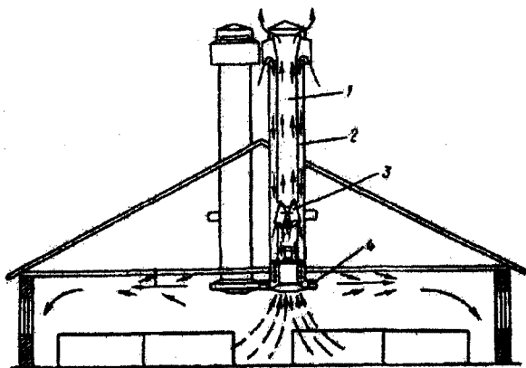
3.3.4-rasm. PVU-so'ruvchi –haydovchi qurilmasi: 1-chiqaruvchi kanal; 2-halqali kirituvchi kanal; 3-aralashtiruvchi zaslonka; 4-tarqatgich.
