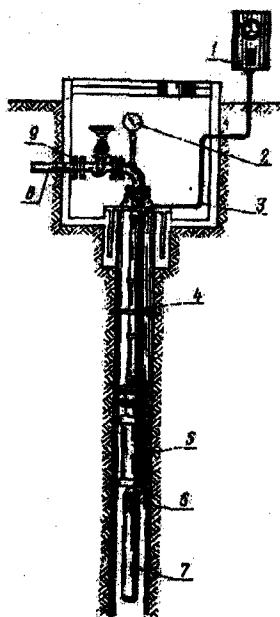
3.2.9-rasm. Cho'ktirmali suv nasosining artezian quduqqa o'rnatilish sxemasi: 1-boshqarish stansiyasi; 2-monometr; 3-elektr kabeli; 4-suv ko'tarish trubasi; 5-nasos; 6-filtr; 7-elektr dvigateli; 8-qoplama trubasi; 9-zadvijka.
