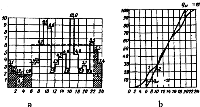
3.2.4. Fermada suv sarflanishining va suv nasosining ishlash grafigi: a-zinapoyali (suv sarflanishini to'g'ri chiziq, nasosning soat 6 dan 20 gacha ishlashi punktirli chiziq); b-integralli; 1-kunlik suv sarfi; 2-nasosning soat 6 dan 20 gacha ishlash grafigi.
