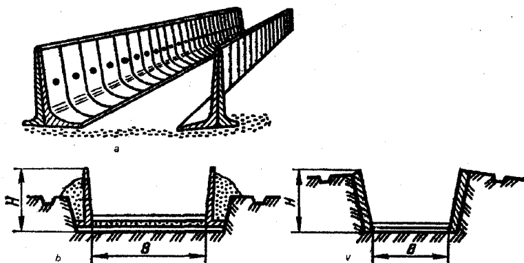
2.1.10-rasm. Silos transheyalari: a -yer ustida; b -yarim ko'milgan; v -ko'milgan; H -transheya balandligi; V -transheya kengligi.
