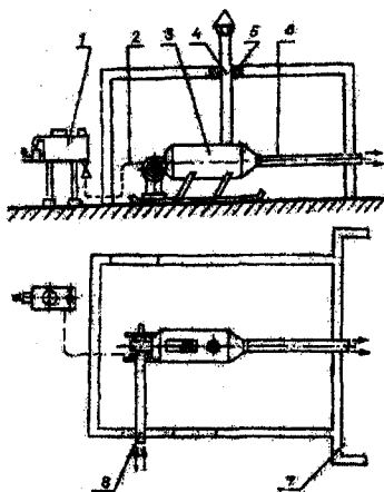
3.3.6-rasm. Issiqlik generatorlari ni chorvachilik binolarida o'rnatish sxemasi:
