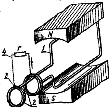
4.1.2 - rasm. Bir fazali o'zgaruvchan tok genegatorining ishlash prinsipi:
