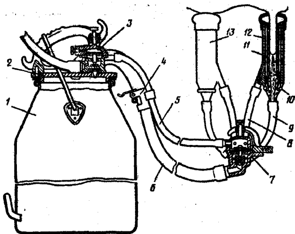
3.6.2-rasm. Sut sog'ish apparatining umumiy tuzilishi:
