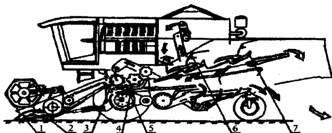
2.1.7 - rasm. "Dominator" kombayni texnologik ish jarayonining sxemasi: 1-boshqoq ko'targich taroqlari; 2-avtokontur sirpangichi; 3-tezlash-tirish barabani; 4-yanchish barabani; 5-tishli segment; 6-sozlanuvchan fartuk; 7-somon elagich klavishasining uzaytirgichi;
