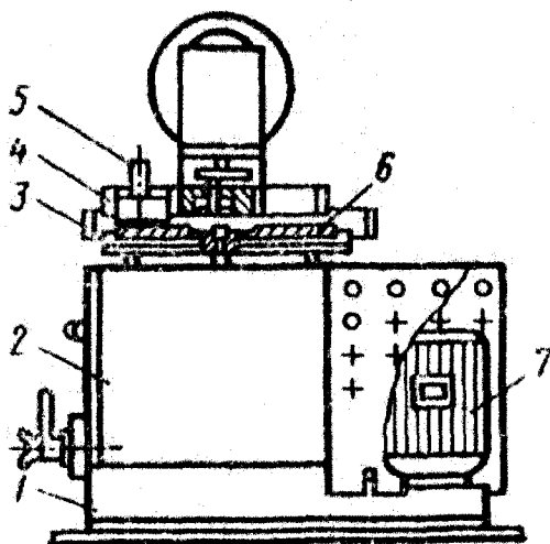
3.8.5-rasm. PZN-60 charxlash yarim avtomati: 1-rama; 2-reduktor; 3-kojux; 4-oboyma; 5-ushlagich; 6-charxlash diski; 7-elektr dvigateli.
