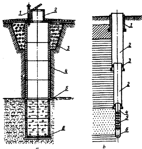
3.2.1-rasm. Shaxtali (a) va trubali (artezian) qurilmalarning sxemasi: a-shaxtali: 1-ventilyasiya trubasi; 2-qopqog'i; 3-loyly tayanch; 4-qoplama; 5-suv olish qismi; b-trubali: 1-konduktor; 2-qoplama trubalar; 3-salniklar; 4-filtrning ustki trubasi; 5-filtrli truba; 6-filtrning tindirgichi.
