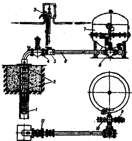
3.2.13. VU-10-80 suv qurilmasi: 1-nasos; 2-oraliq tutashtirgichlar; 3-boshqarish stansiyasi; 4-flya- nets; 5-teskari klapan; 6-suv truba- si; 7-idroakkumulyator; 8-kran; 9-yong'in krani; 10-saqlovchi kla- pan; 11-zadvijka.
