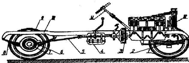
1.3.4 - rasm. Avtomobilning asosiy mexanizmlari va yig'ma qismlarining joylashishi: 1-boshqariluvchi g'ildirak; 2-oldingi osma; 3-tishlashish muftasi; 4-uzatmalar qutisi; 5-kardanli uzatma; 6-bosh uzatma; 7-differensial; 8-ketingi osma; 9-yetakchi g'ildirak; 10-rama; 11-boshqaruv ruli; 12-dvigatel.
