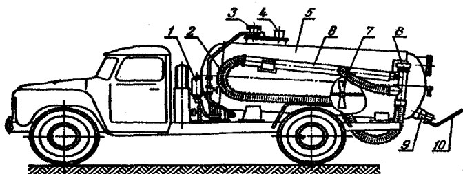
1.4.1- rasm. RJU-3,6 markali shaltoq sochgich - sisterna:
