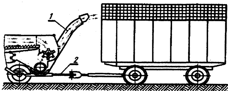
2.1.8-rasm. PUN-5 moslamasi yordamida somonni maydalab yig'ishtirish sxemasi: 1-trubali yo'lak; 2-avtopritsep; 3-telejka.
