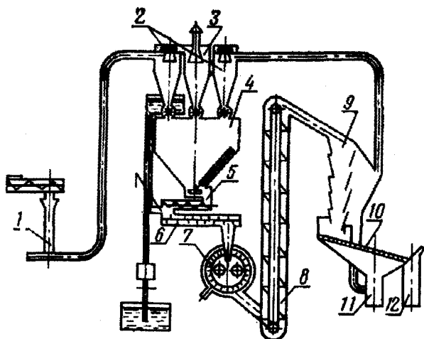
2.1.13 - rasm. OGM-1,5 qurilmasida vitaminli o't unidan donador(granula) tayyorlash sxemasi:
