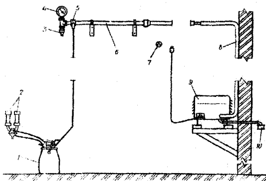
3.6.7-rasm. AID-1 sut sog'ish agregati. 1-sog'ish chelagi;
