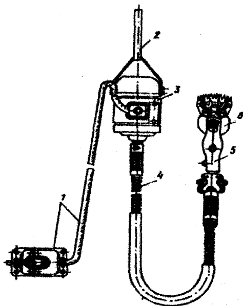
3.8.3-rasm. ESA-1D jun qirqish agregati:
