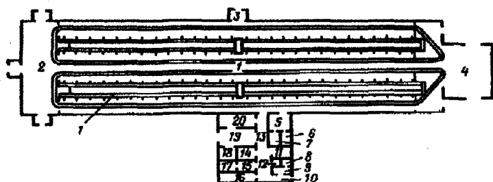
3.1.6-rasm. 200 bosh sigirga mo'ljallangan sigirxonaning plani: 1-sigirlar boyloqli turadigan maydon; 2-oziglantirish yo'lagi; 3-sigirlarni sun'iy qochirish laboratoriyasi; 4-sutxona; 5-vakuum nasos; 6-yuvish xonasi; 7-vetlaboratoriya.
